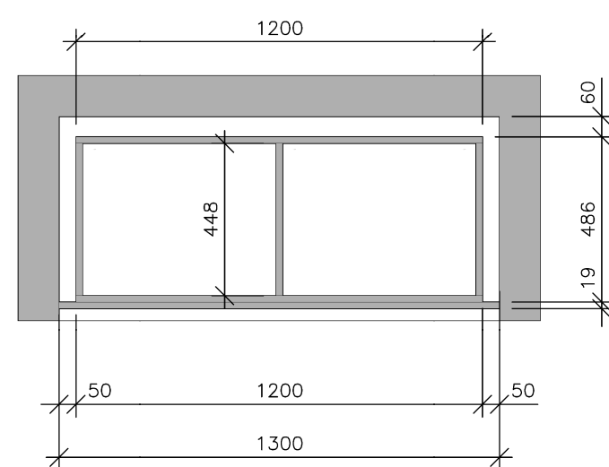
Vue Socle
