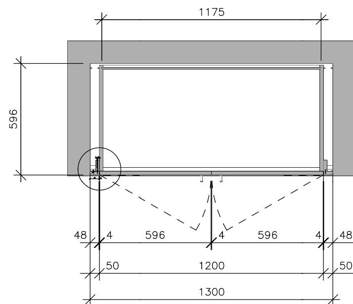
Détail Fabrication 01
